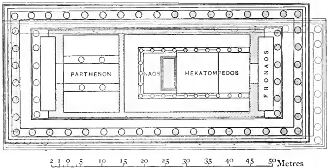
FIG. 62.—PLAN OF THE PARTHENON.
